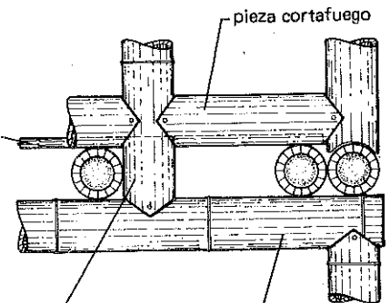
a ALZADA
