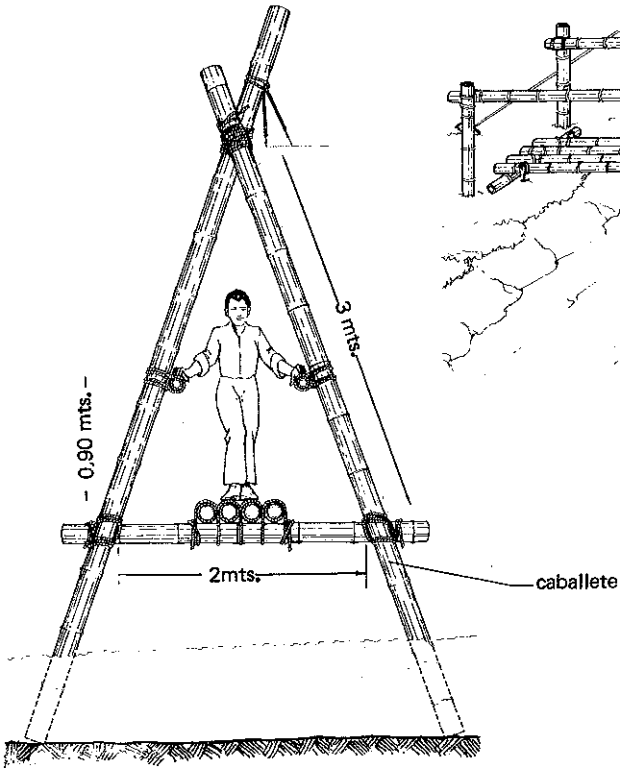
SECCION TRANSVERSAL
