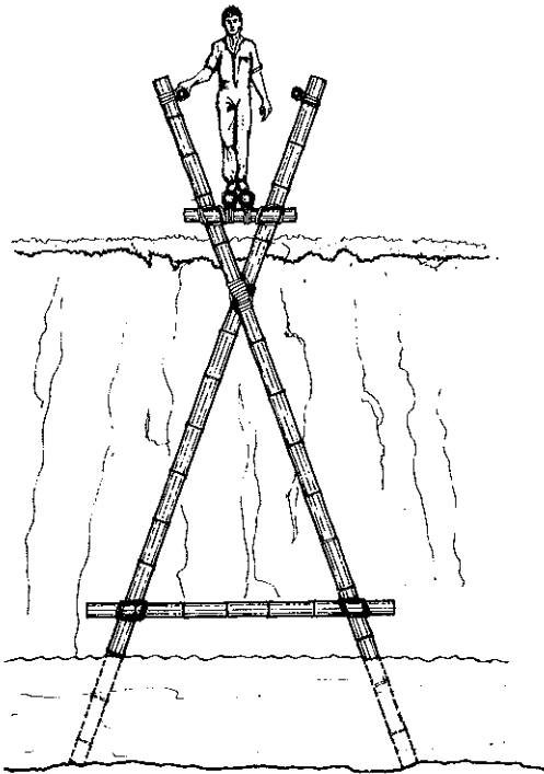
SECCION TRANSVERSAL
