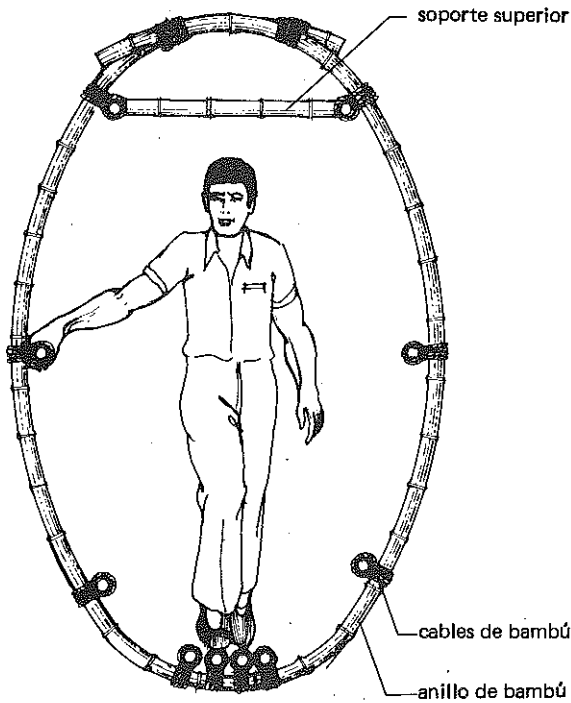
SECCION TRANSVERSAL
