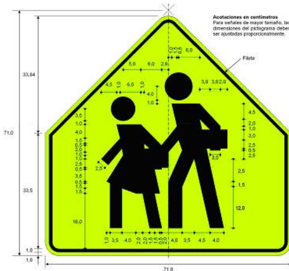
FIGURA 28.- Señal preventiva SP-33 "Escolares" de 71 x 71 cm
