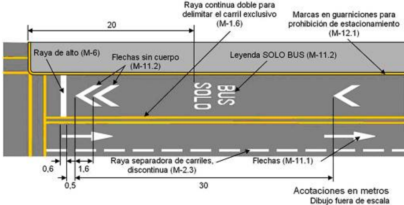
FIGURA 4.- Marcas para delimitar un carril en contrasentido
