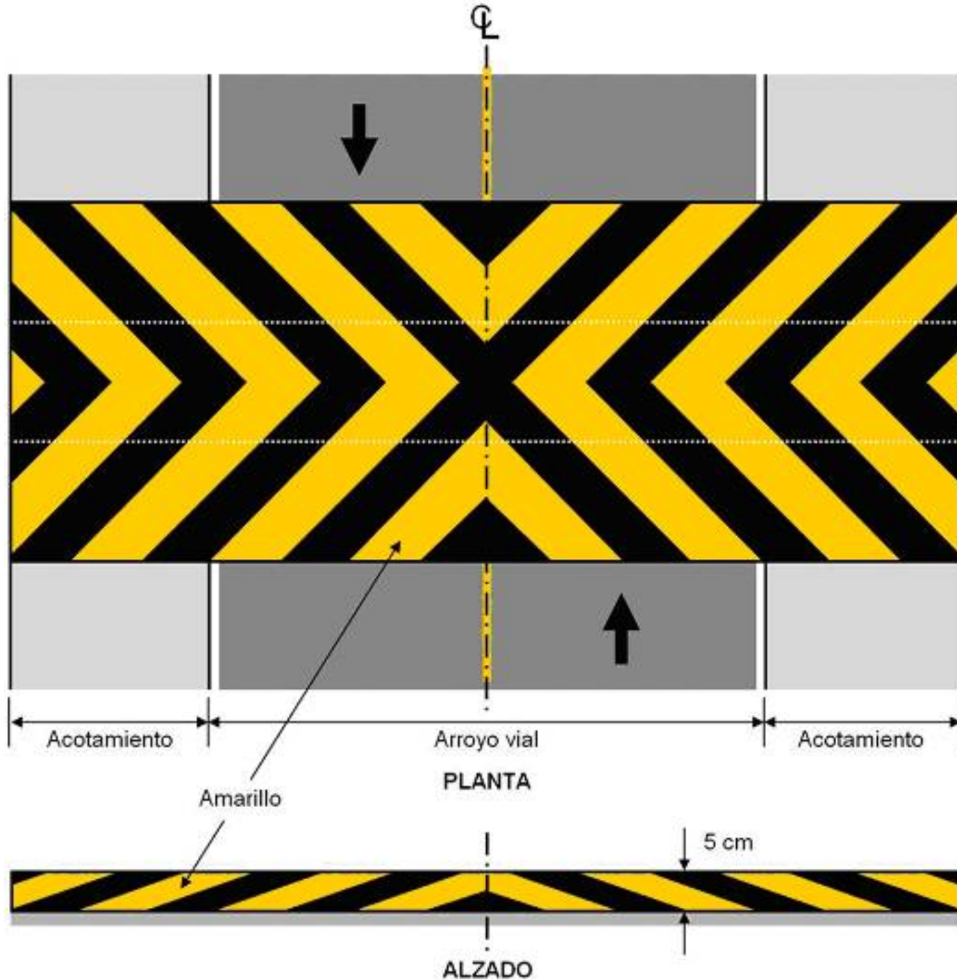
FIGURA 27.- Color de los reductores de velocidad (RV)
