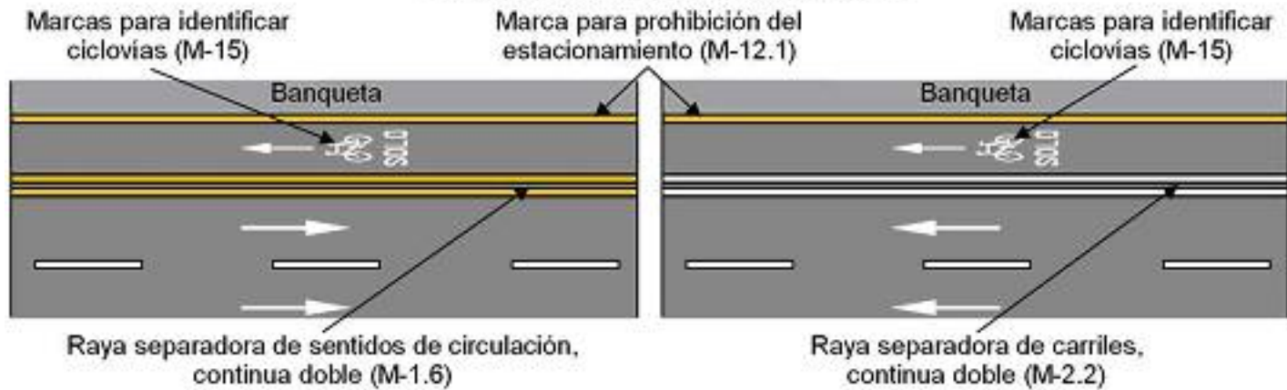
FIGURA 24.- Marcas para delimitar ciclovías
