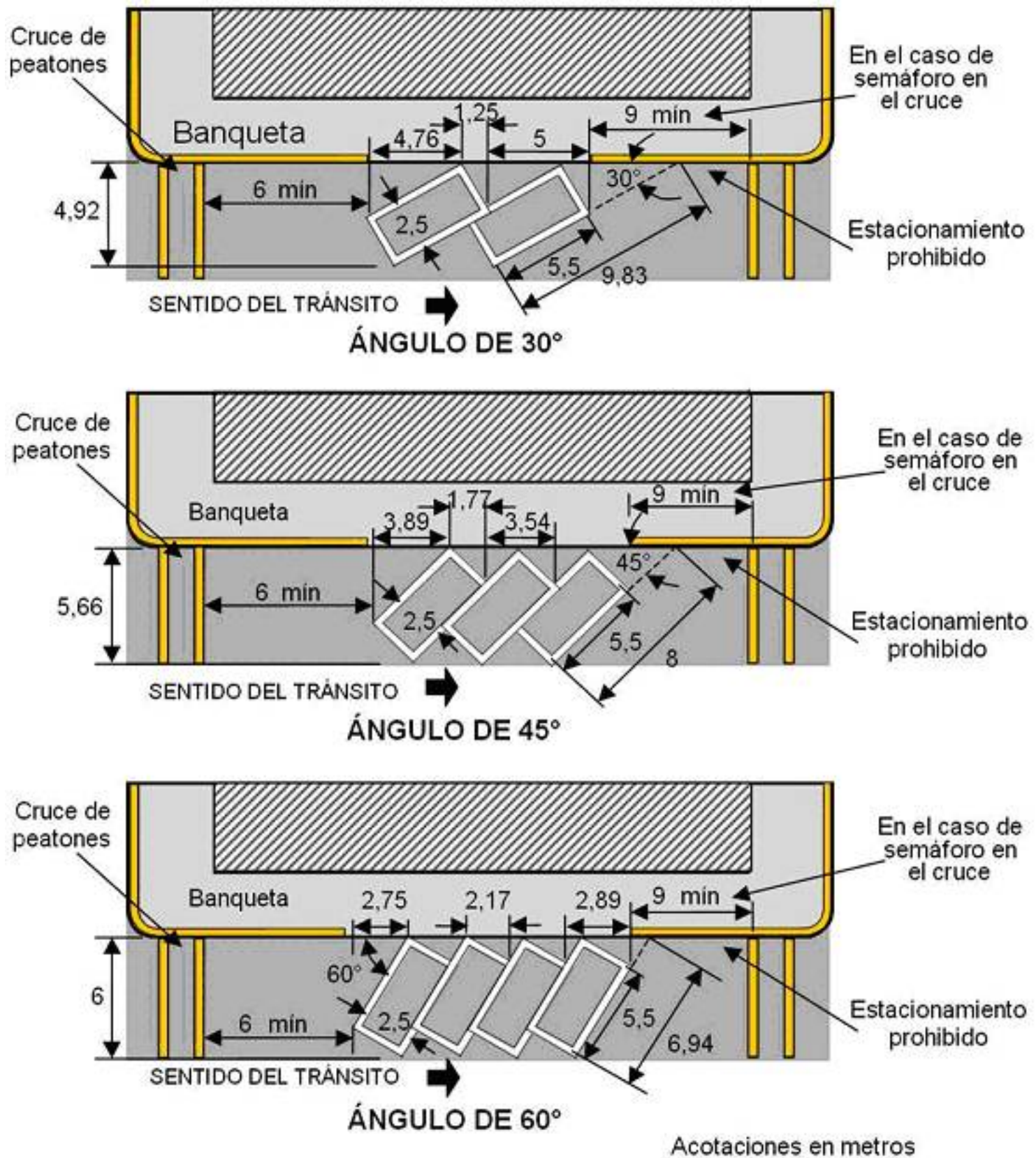
FIGURA 16.- Marcas para estacionamiento en batería
