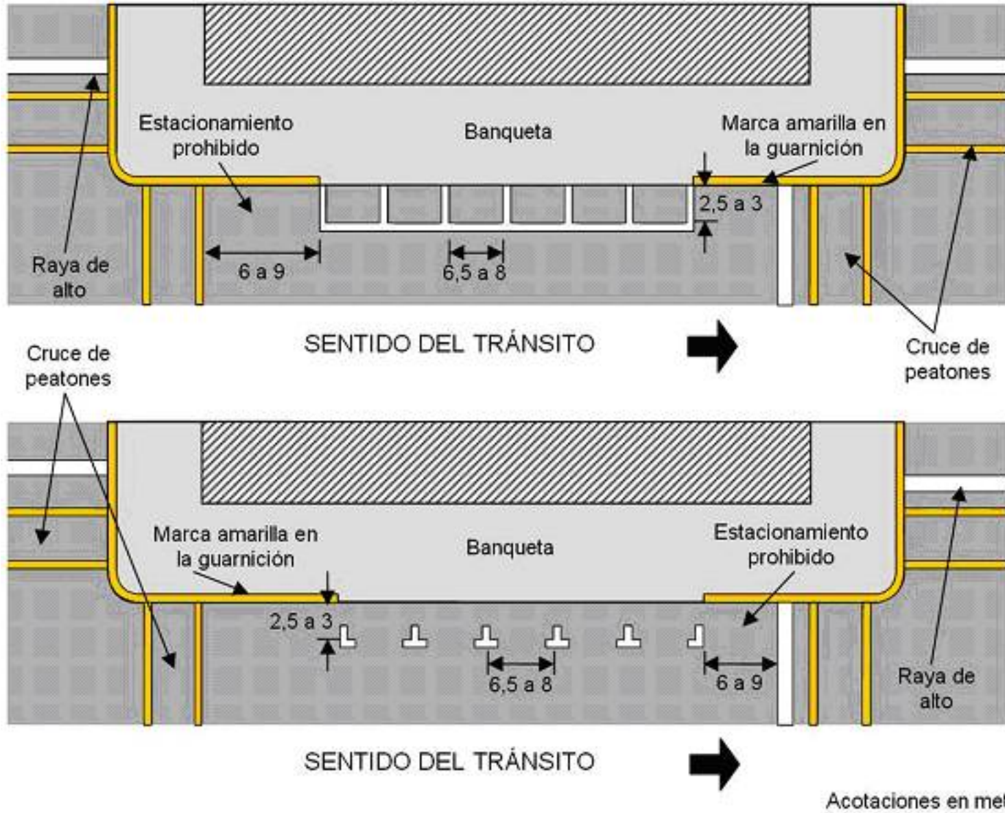
FIGURA 15.- Marcas para estacionamiento
