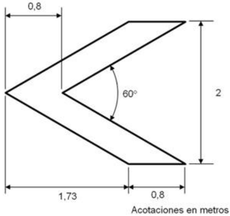
FIGURA 19.- Flechas sin cuerpo
