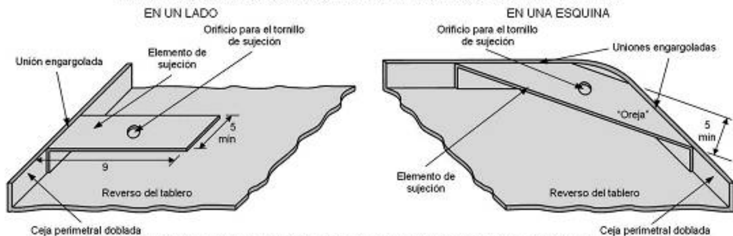
FIGURA 34.- Disposición de los elementos de sujeción en señales bajas
