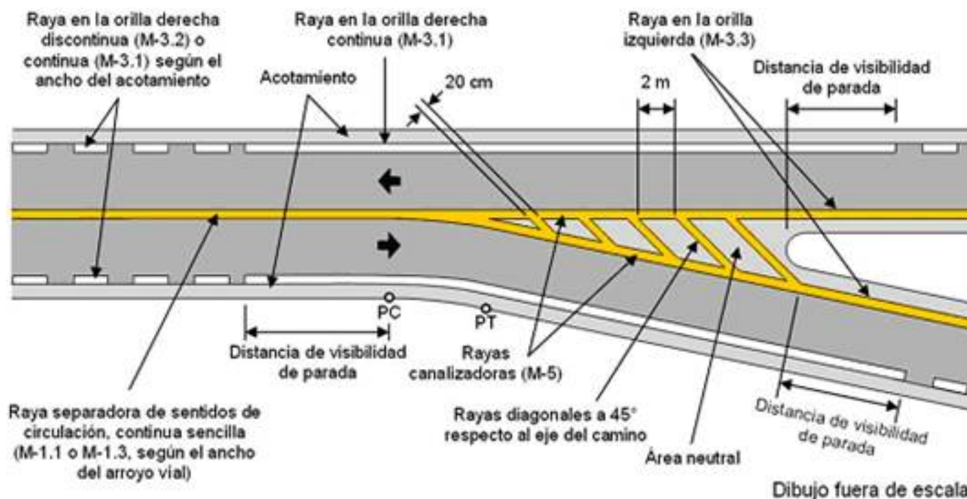
FIGURA 9.- Rayas canalizadoras
