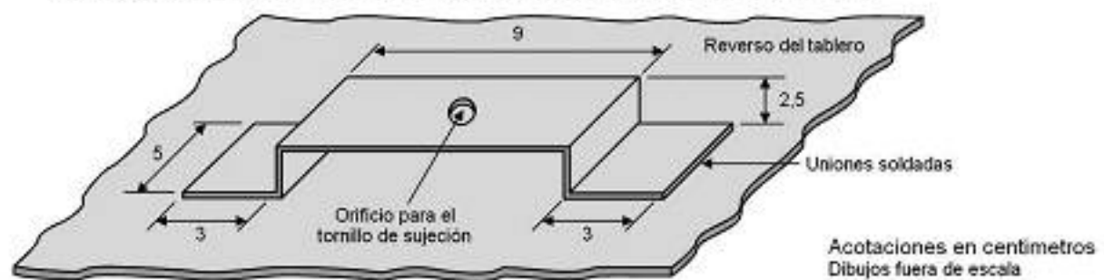
FIGURA 35.- Elementos de sujeción para señales bajas
