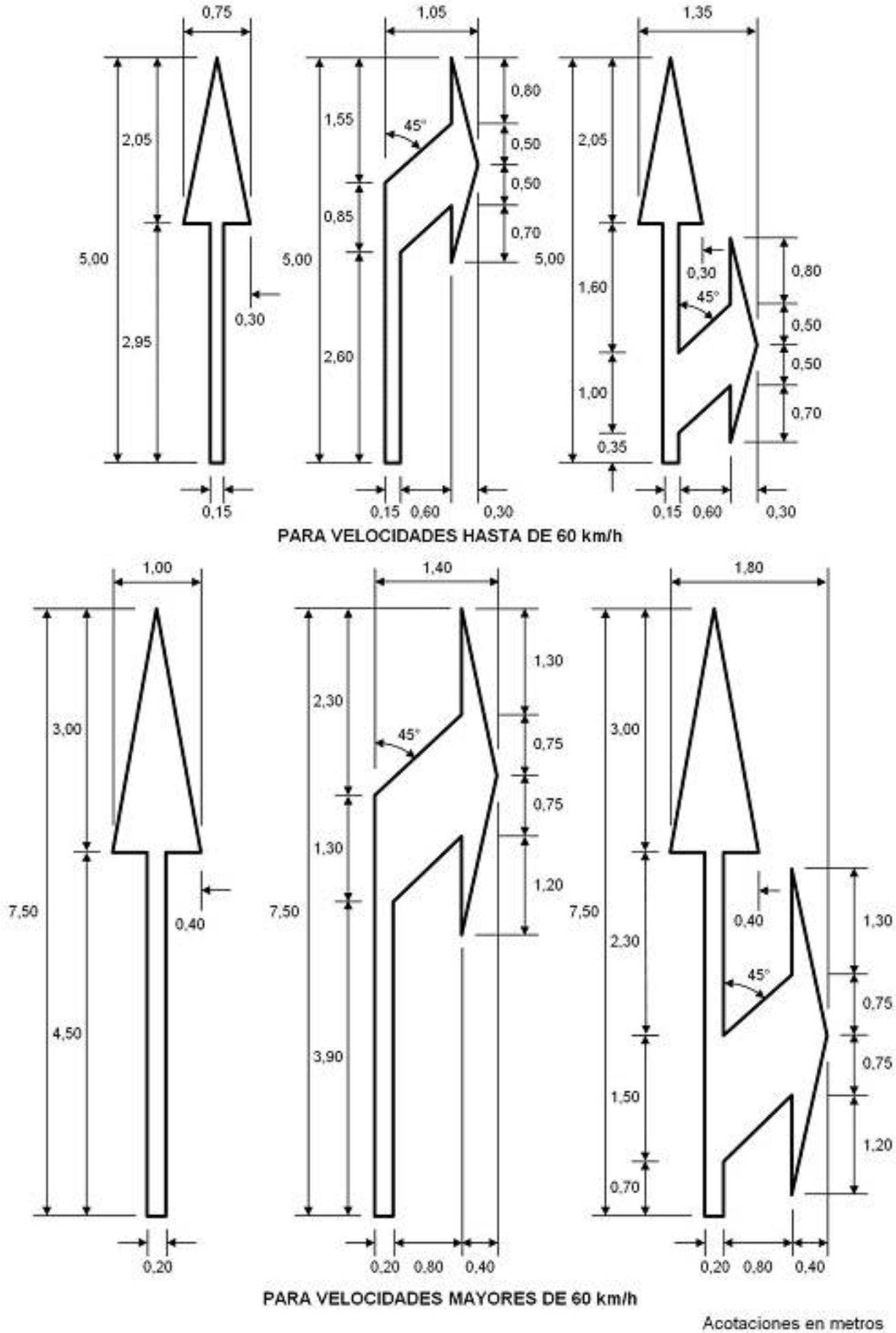
FIGURA 18.- Flechas de dirección para carriles
