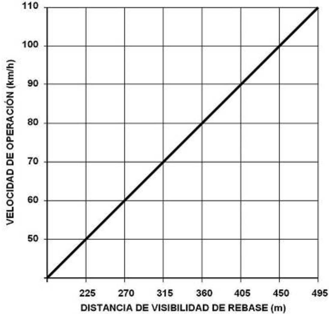
GRÁFICA A1.- Distancia de visibilidad de rebase
