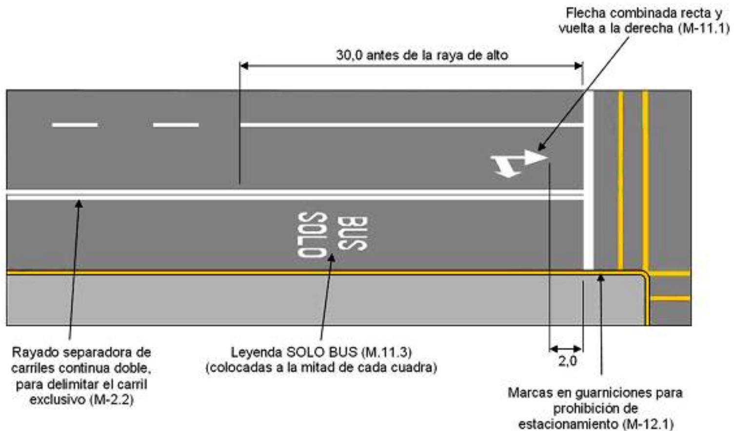
FIGURA 8.- Marcas para delimitar un carril exclusivo
