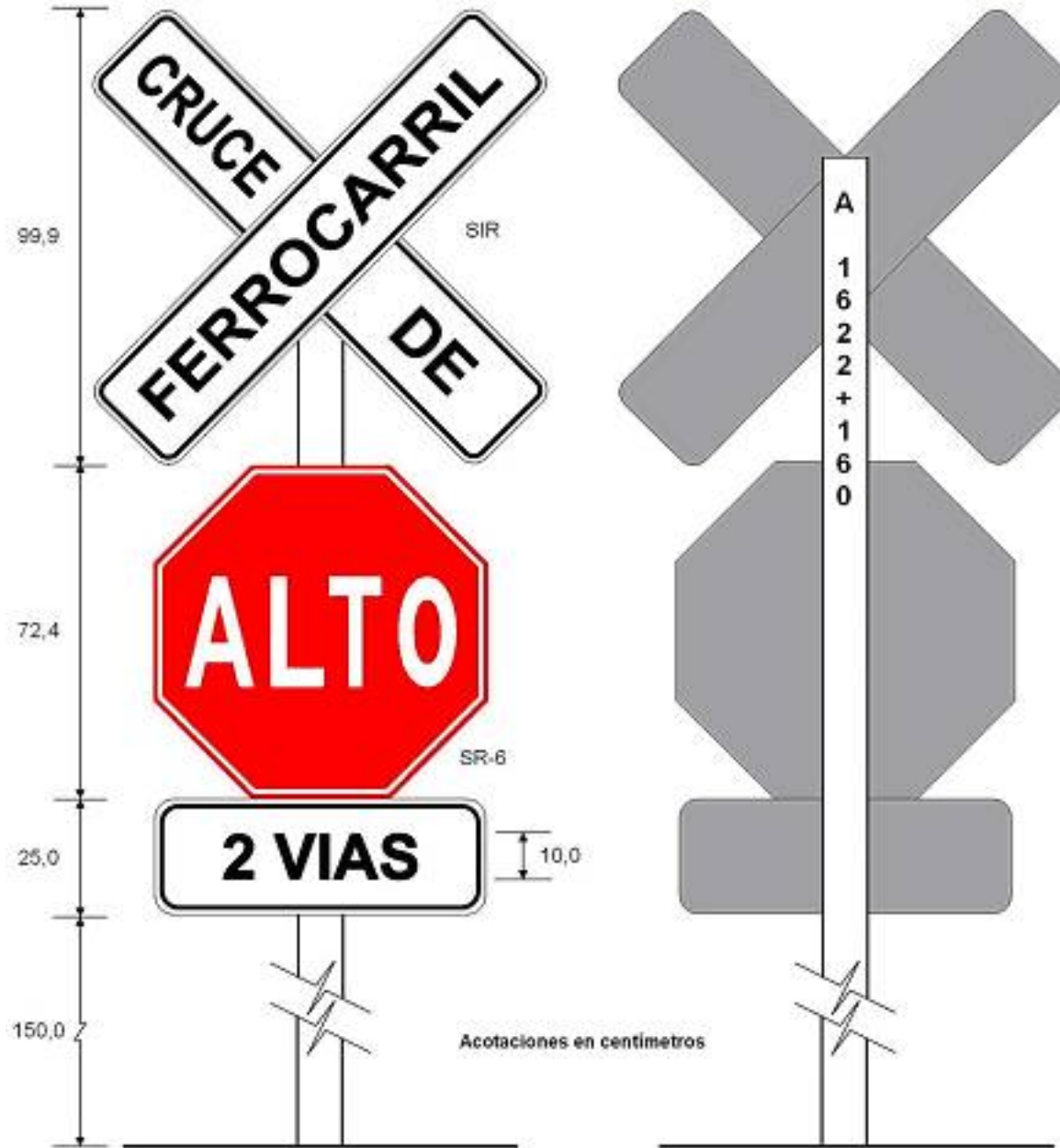
FIGURA B7.- SIR "Cruce de ferrocarril"
