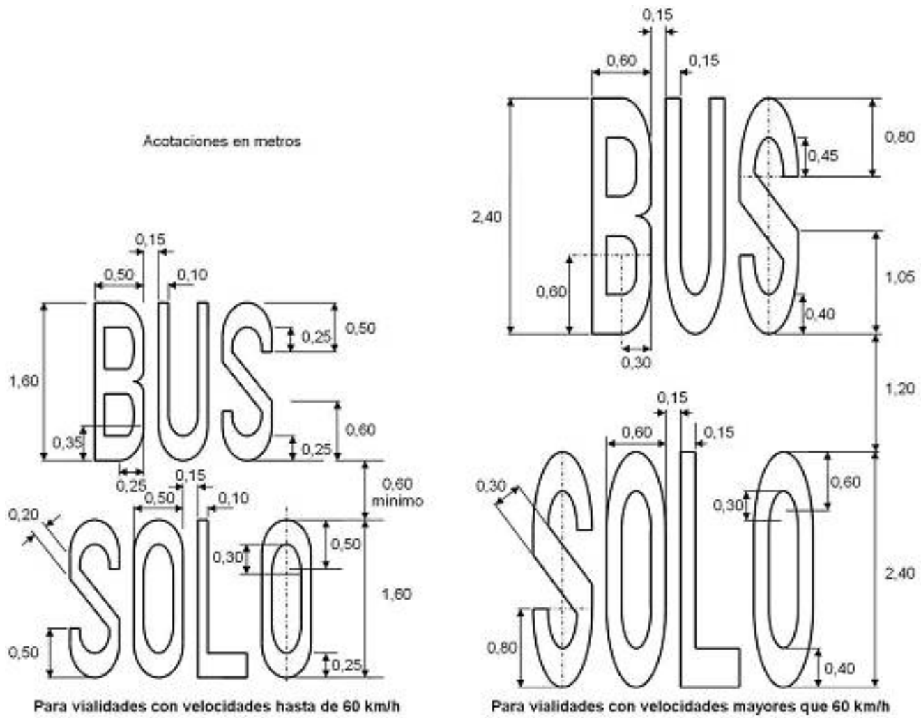
FIGURA 20.- Leyenda SOLO BUS
