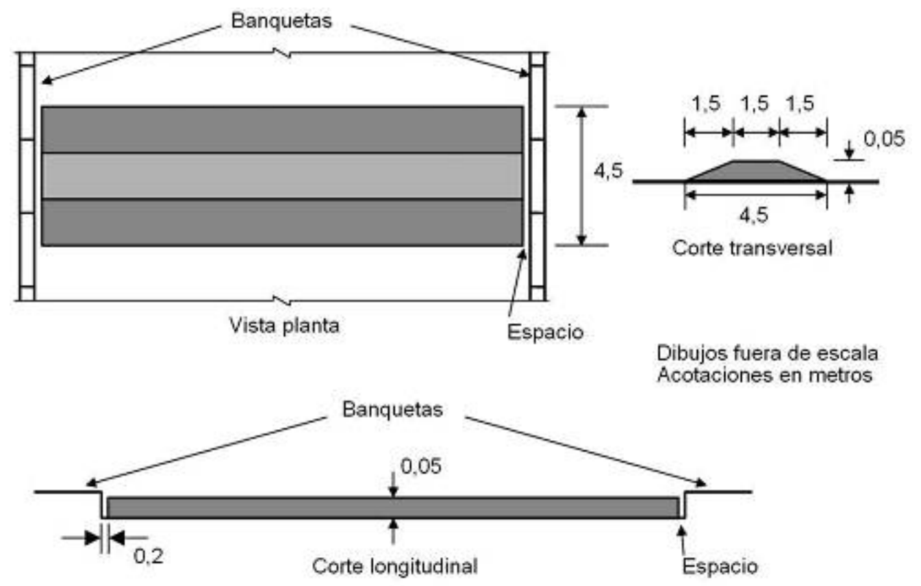
FIGURA 26.- Reductor de velocidad (RV)
