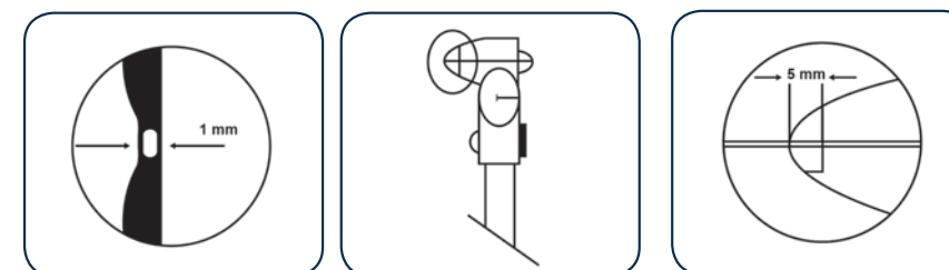
Fig. 2. Sección transversal de tres perfiles principales típicos y espesor mínimo en las clases A,B y C.
