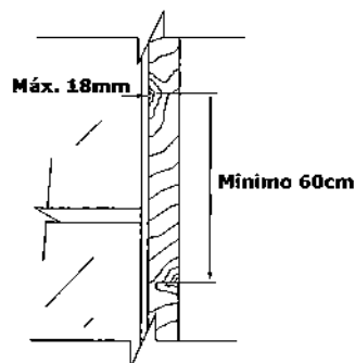
Tamaño y separación de nudos en ventanas de madera
